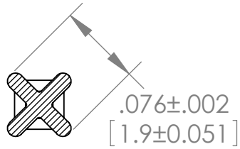
SECTION A-A SCALE 8 : 1
