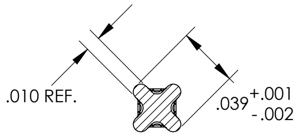
SECTION A-A SCALE 16 : 1
